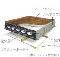
〈ボイドスラブ概念図〉
