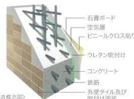
〈外壁構造概念図〉
