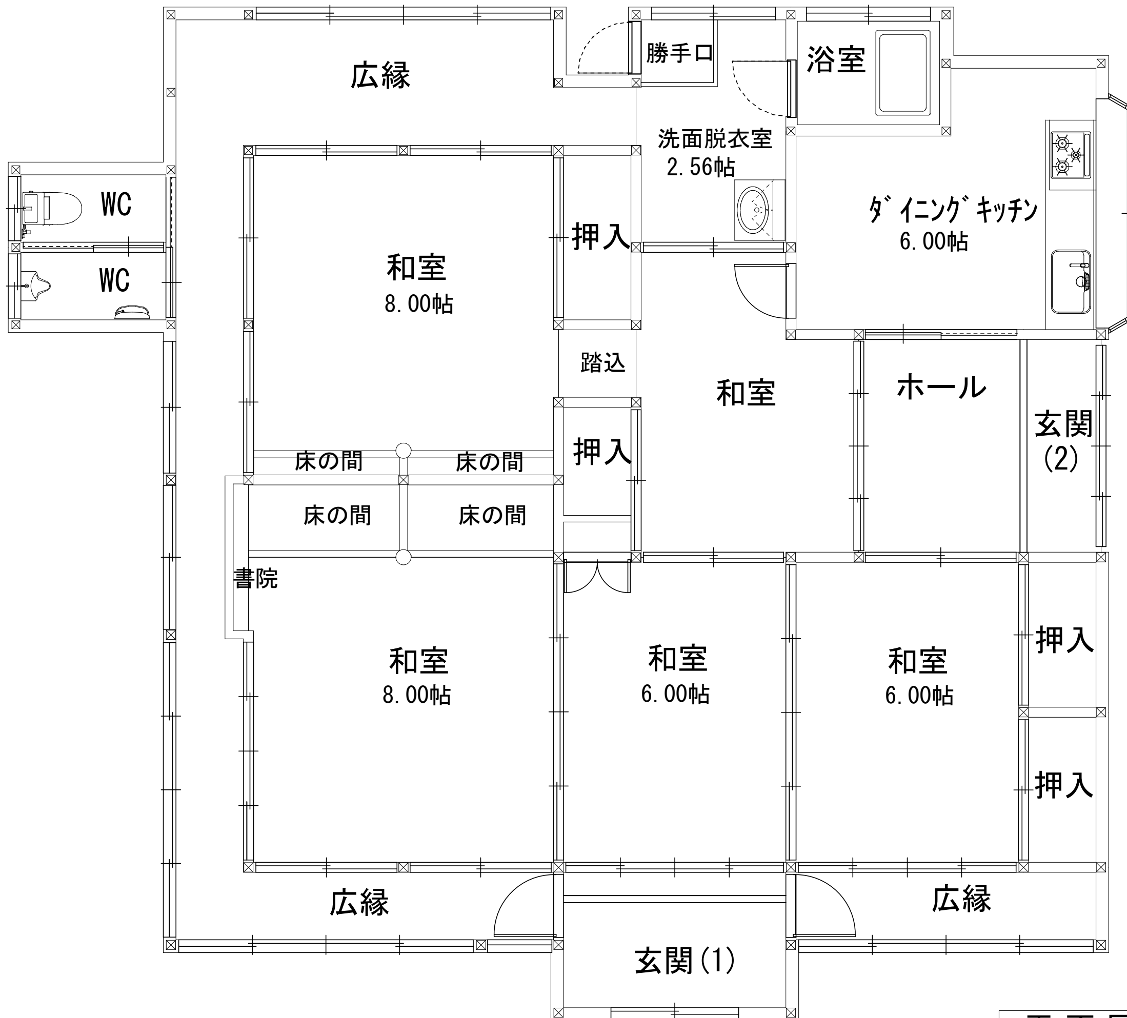
平面図 S = 1 / 50
